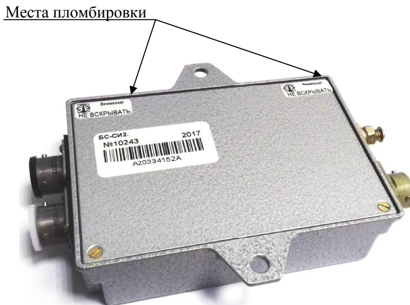
Рисунок 2 - Схема пломбировки от несанкционированного доступа
