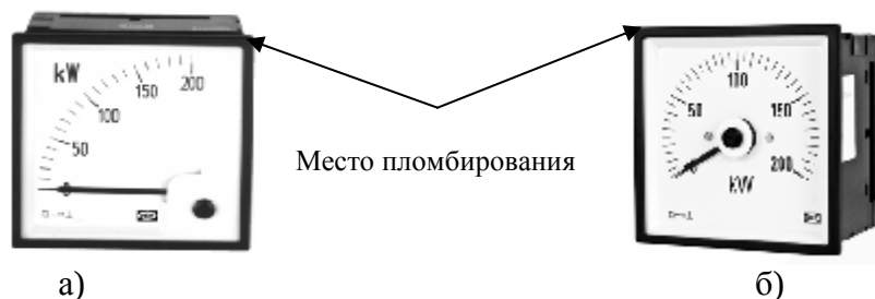
Рисунок 1. - а) внешний вид измерителя с углом перемещения указателя 90^\circ ; б) внешний вид измерителя с углом перемещения указателя 240^\circ .
