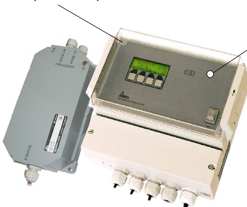
Рисунок 4 - Схема пломбировки от несанкционированного доступа и схема нанесения знака поверки на преобразователи с выносным входным усилителем
