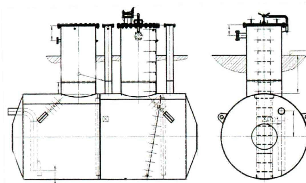
Рисунок 2 - Эскиз резервуаров РГС-12,5 №№ 6651, 6652
