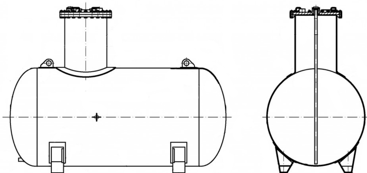
Рисунок 1 - Общий вид эскиза резервуаров РГС-12,5
