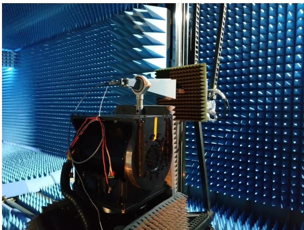
Рисунок 2 – Общий вид ОПУ с установленной измеряемой антенной и сканера с установленной антенной-зондом
