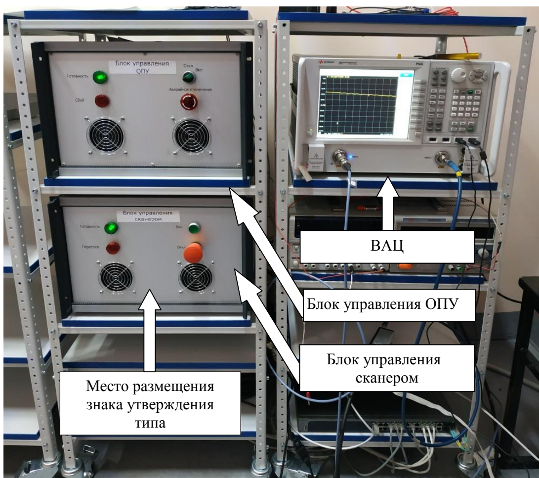
Рисунок 4 – Общий вид векторного анализатора цепей, блока управления сканером и блока управления ОПУ комплекса с указанием места размещения знака утверждения типа
