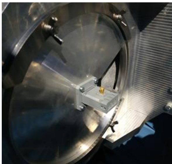
Рисунок 3 – Общий вид крепежа антенны-зонда и ПЭВМ
