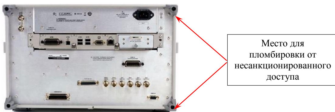
Рисунок 6 – Задняя панель ВАЦ с указанием места пломбировки от несанкционированного доступа
