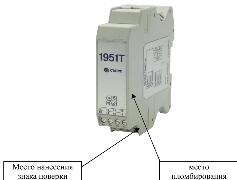
Рисунок 2 – Внешний вид модуля СИЭЛ–1951Т
