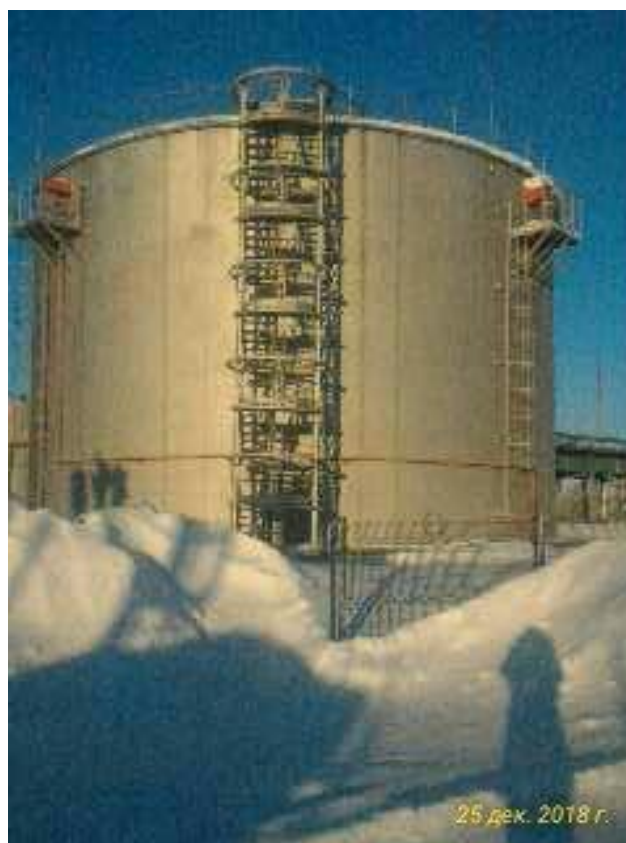
Рисунок 3 - Общий вид резервуара вертикального стального цилиндрического РВС-3000
