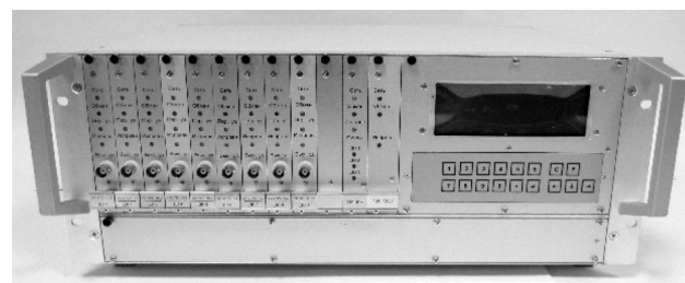
Рисунок 7 - Аппаратура измерения роторных вибраций ИВ-Д-СФ-3М
