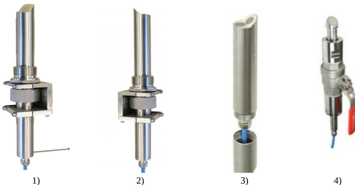
Рисунок 5 - Общий вид 1) трубного датчика скорости длиной 30см (тип POA), 2) комбинированного трубного датчика скорости со встроенным ультразвуковым датчиком уровня длиной 30 см (тип POA), 3) комбинированного трубного датчика скорости длиной свыше 30 см (тип POA), 4) трубного датчика с шаровым краном и приварной насадкой (тип CSM)
