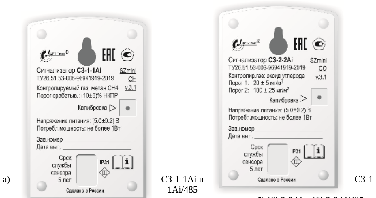
Рисунок 2 - Общий вид сигнализаторов загазованности С3-Аi, вид сзади
