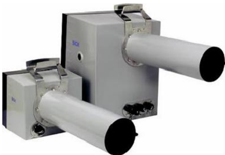
Рисунок 1 – Внешний вид газоанализаторов тоннельных модели VICOTEC320
