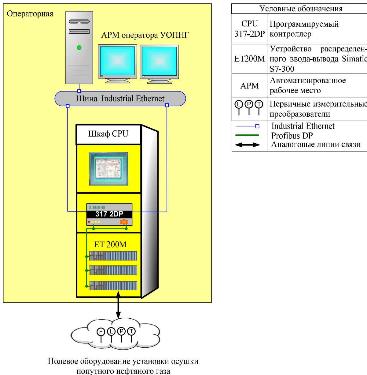
Рисунок 1 - Структурная схема комплекса
