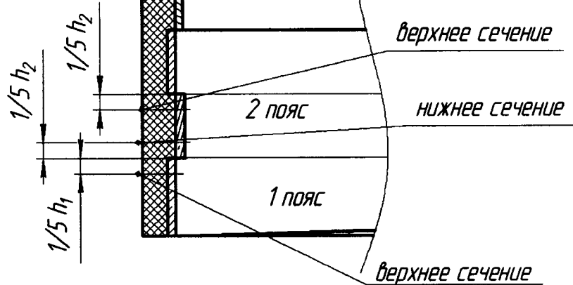
Рисунок А.4 – Схема расположений плоскостей измерений (сечений) внутренних радиусов резервуара
