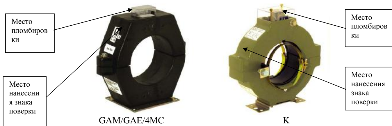
Рисунок 1 – Общий вид трансформаторов тока GAM/GAE/K/4MC.
