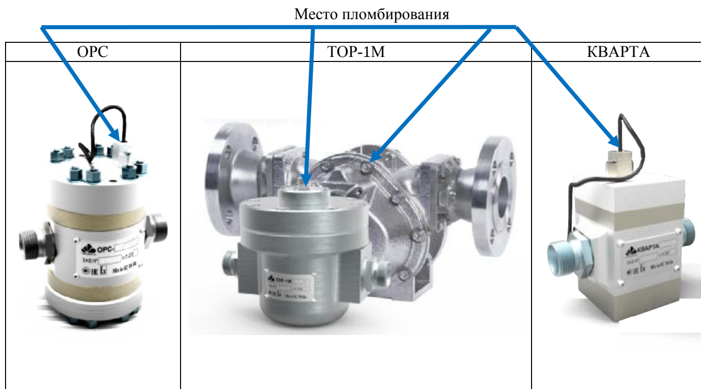
Рисунок 1 – Общий вид и места пломбирования первичного преобразователя расхода
