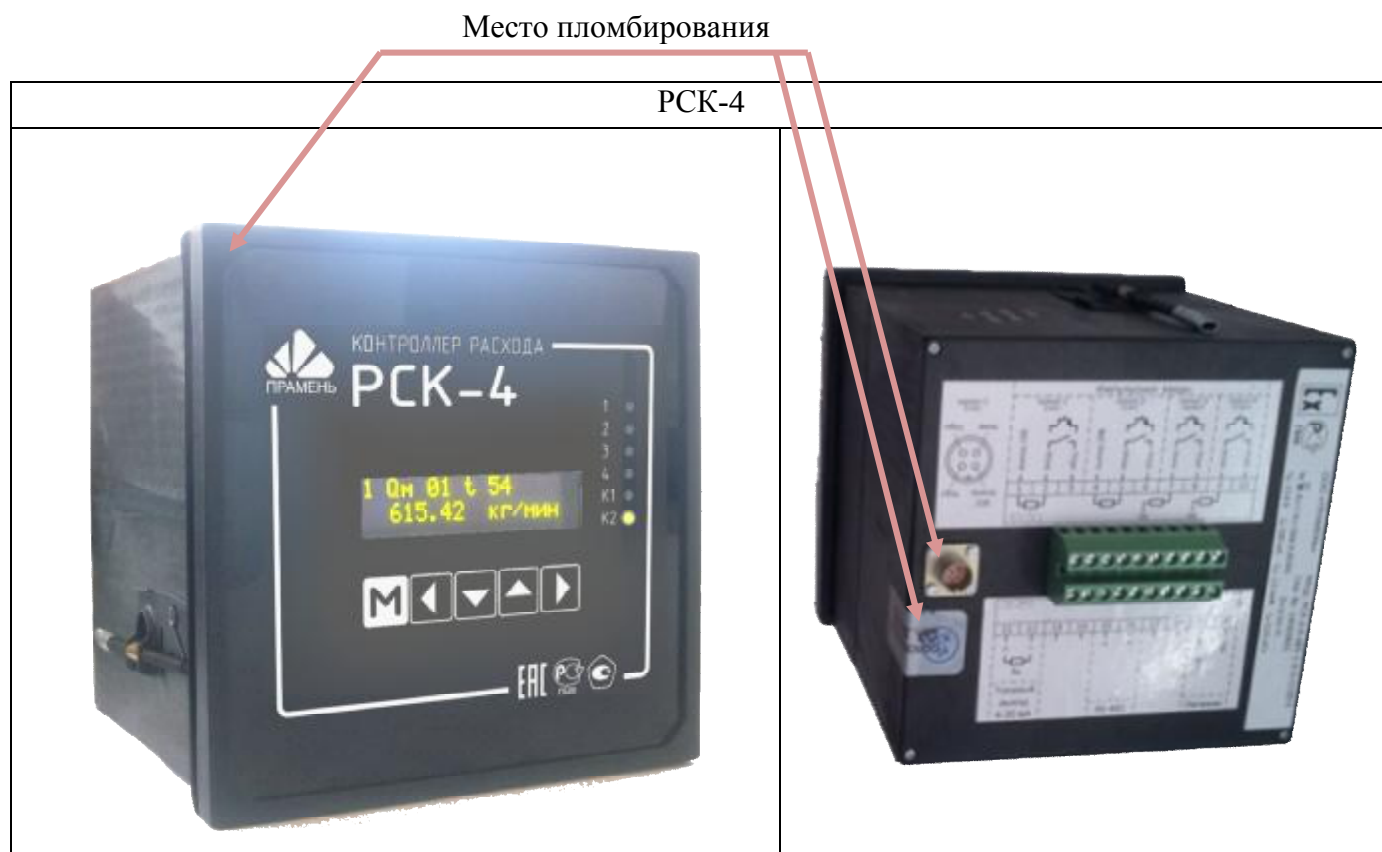
Рисунок 2 – Общий вид и места пломбирования вторичного преобразователя расхода
