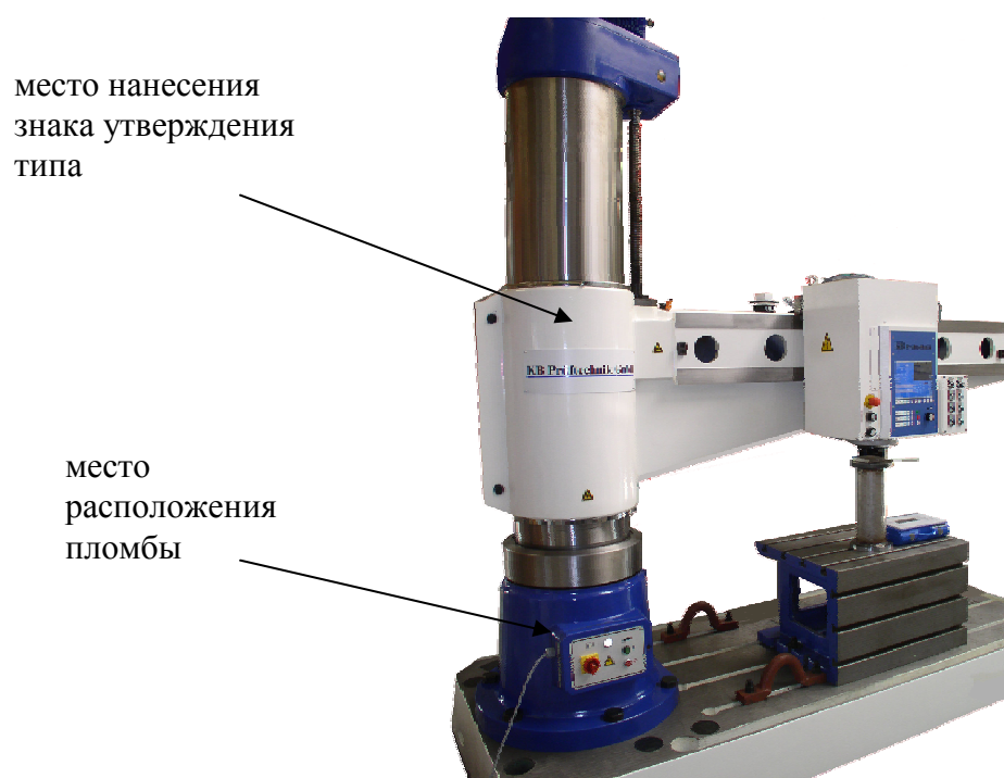
Рисунок 1 – Внешний вид твердомеров
