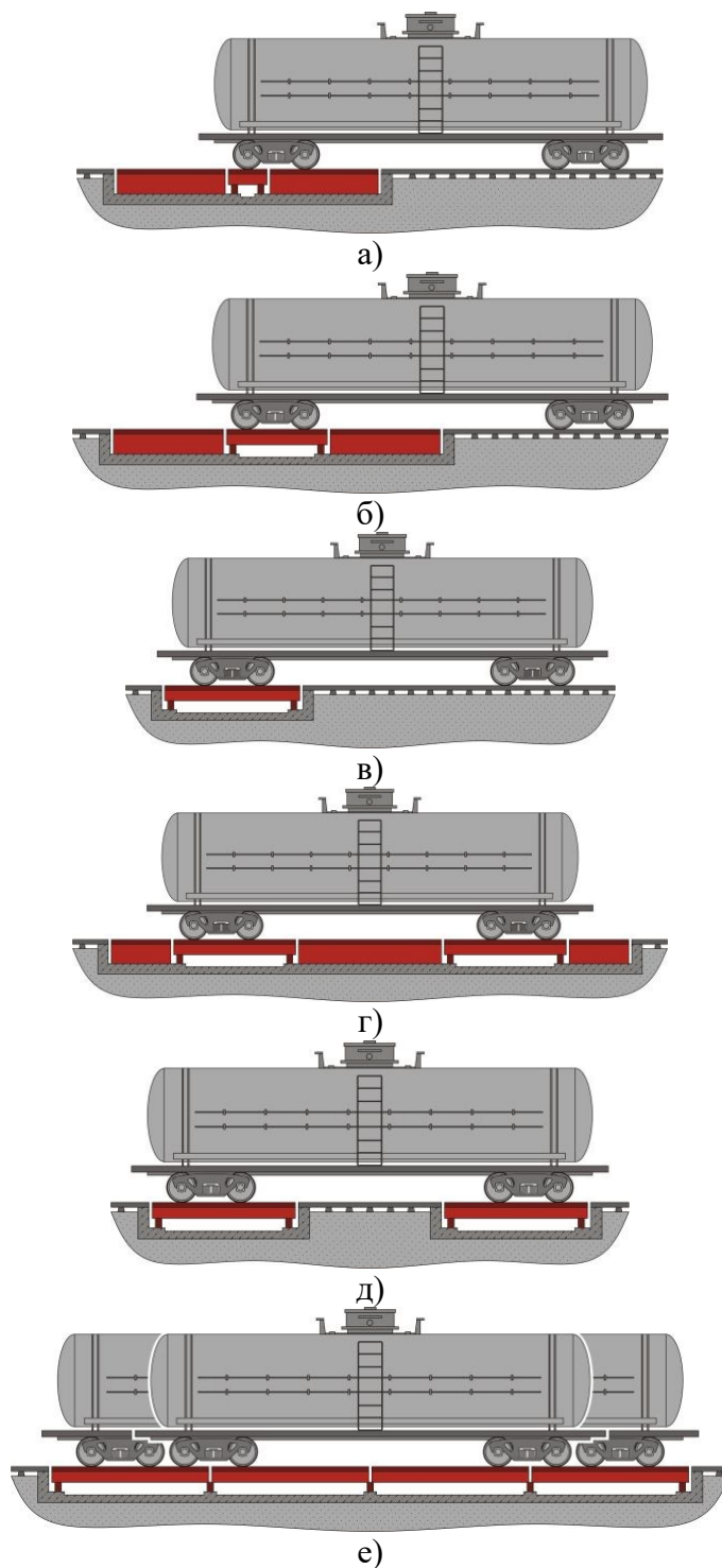
Рисунок 1 Схемы ГПУ весов РД-Д:
