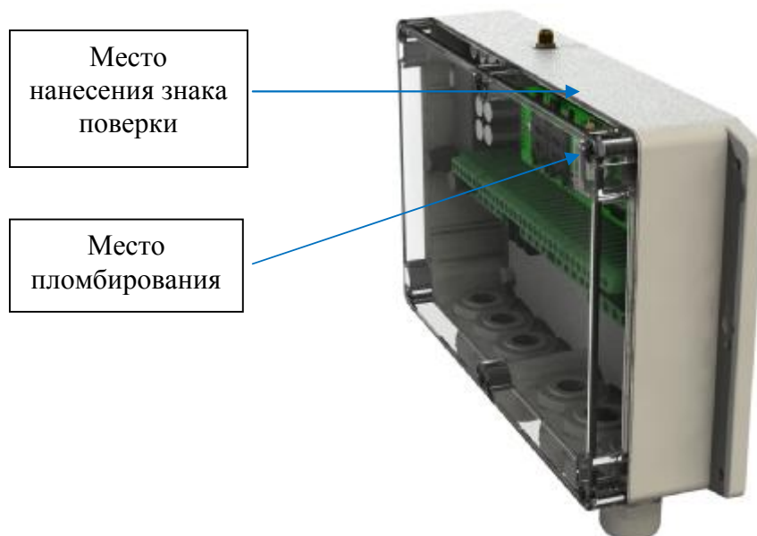
Рисунок 7 - Общий вид исполнения устройств derRTU-P
