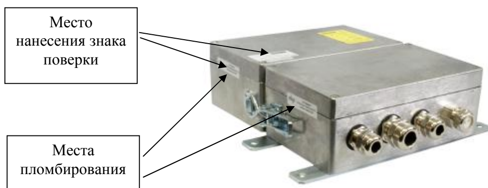
Рисунок 2 - Общий вид полевого исполнения устройств derRTU-ПП
