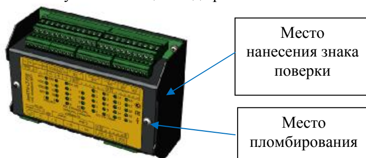
Рисунок 4 - Общий вид крейтового исполнения устройств depRTU-H
