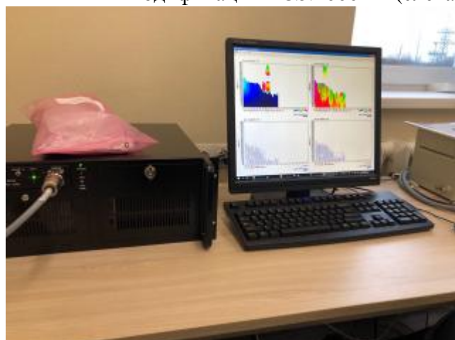
Рисунок 2 – Внешний вид интерфейсного модуля и ПК, смонтированных в едином корпусе (слева). Модуль питания (справа)
