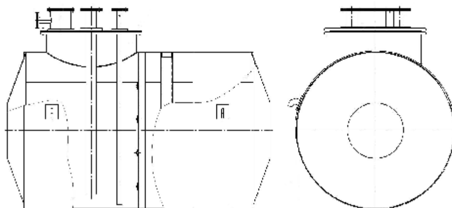
Рисунок 1 – Эскиз резервуаров стальных горизонтальных цилиндрических РГС-50, РГС-60
