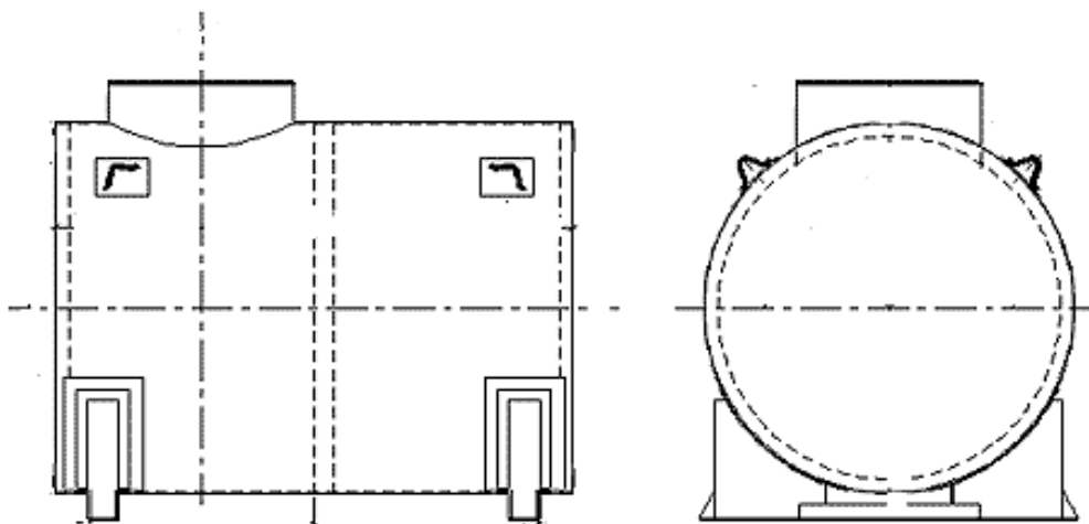
Рисунок 1 – Эскиз резервуара стального горизонтального цилиндрического РГС-25
