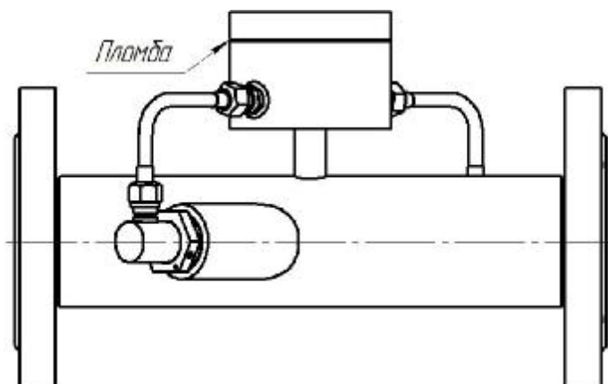
Рисунок 2 - Схема пломбирования
