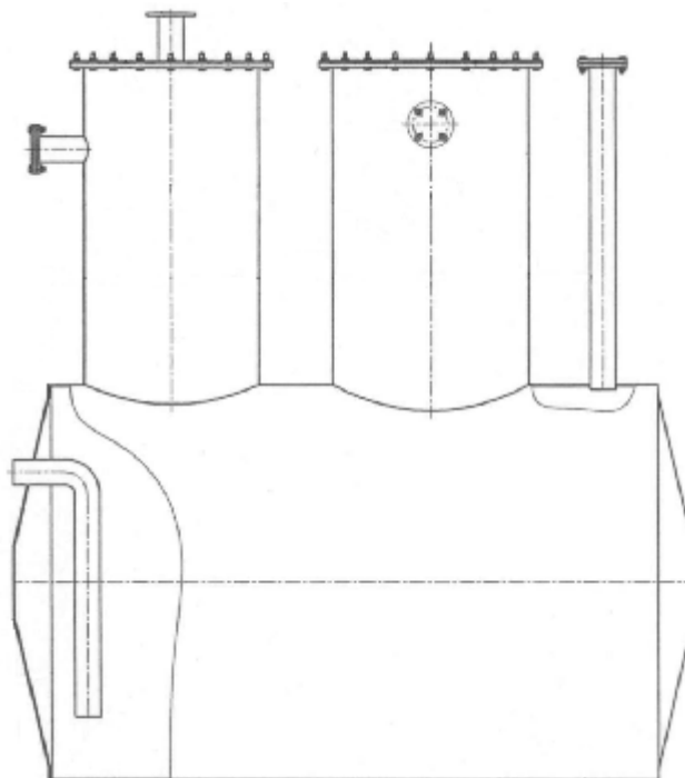
Рисунок 1 – Эскиз резервуара РГС-12,5
