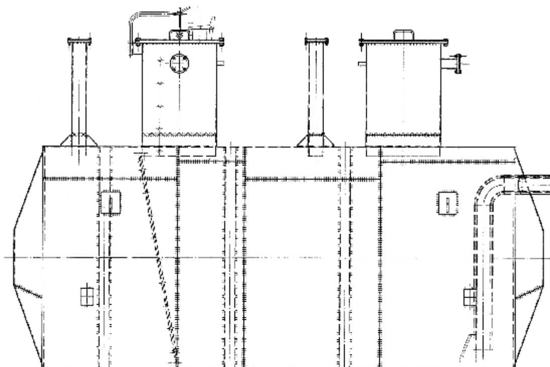
Рисунок 1 – Эскиз резервуаров РГС-25, РГС-40
