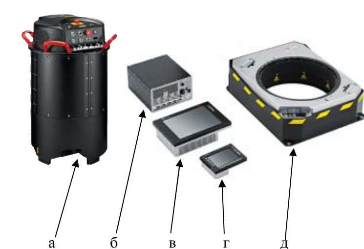
а – сканирующий блок б – блок системного контроллера CC43 в – консоль оператора ОС60 г – дисплей пилота PD60 д – гиростабилизирующая платформа PAV100
