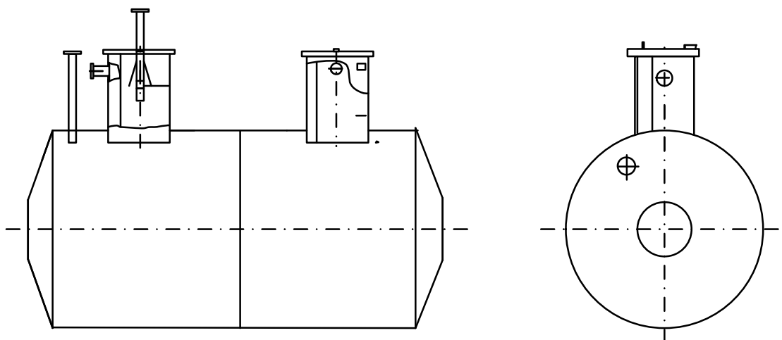
Рисунок 1 – Эскиз резервуара стального горизонтального цилиндрического РГС-25
