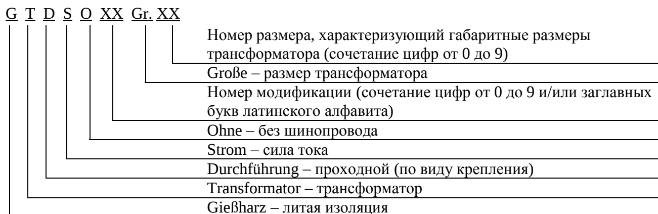
Рисунок 2 – Структура условного обозначения трансформаторов тока GTDS(O)
