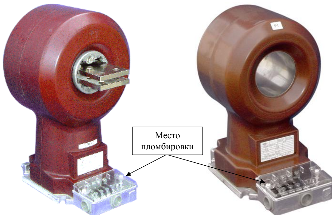
Рисунок 3 – Общий вид трансформаторов модификаций GSS 12, GSS 24, GSS 12 Gr. XX, GSS 24 Gr. XX
