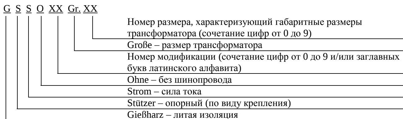
Рисунок 1 – Структура условного обозначения трансформаторов тока GSS(O)
