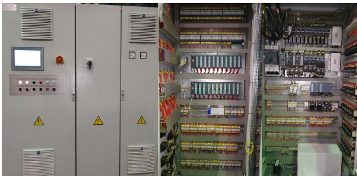
Рисунок 1 – Общий вид щита управления РО55 (ЩУ2)
