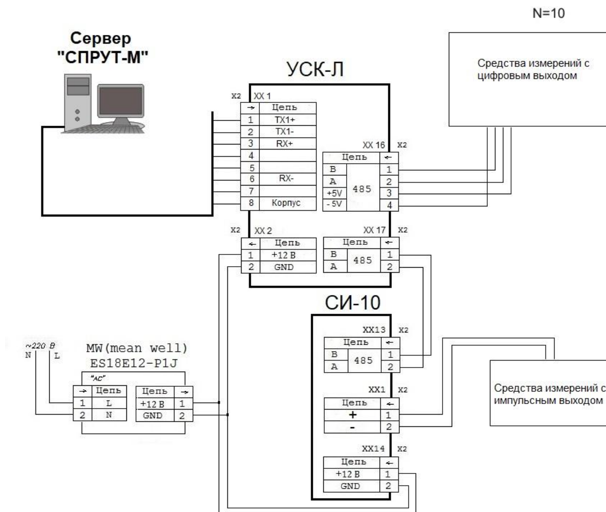
Рисунок 1 – Структурная схема ИВК
