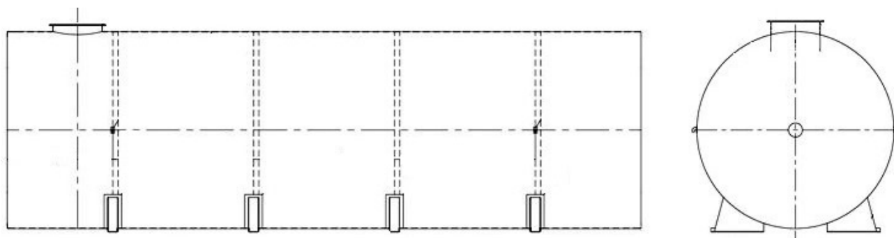
Рисунок 1 – Эскиз общего вида резервуаров стальных горизонтальных цилиндрических РГС-25
