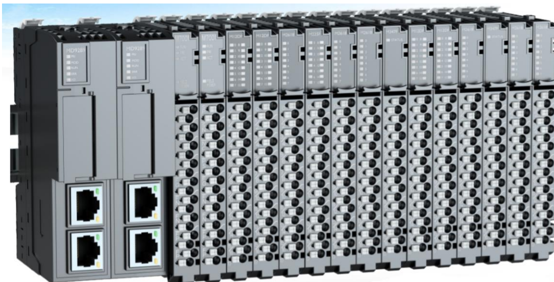
Рис. 4. Общий вид системы распределенного ввода/вывода CREVIS/CYЭP серии М (с поддержкой горячей замены модулей)
