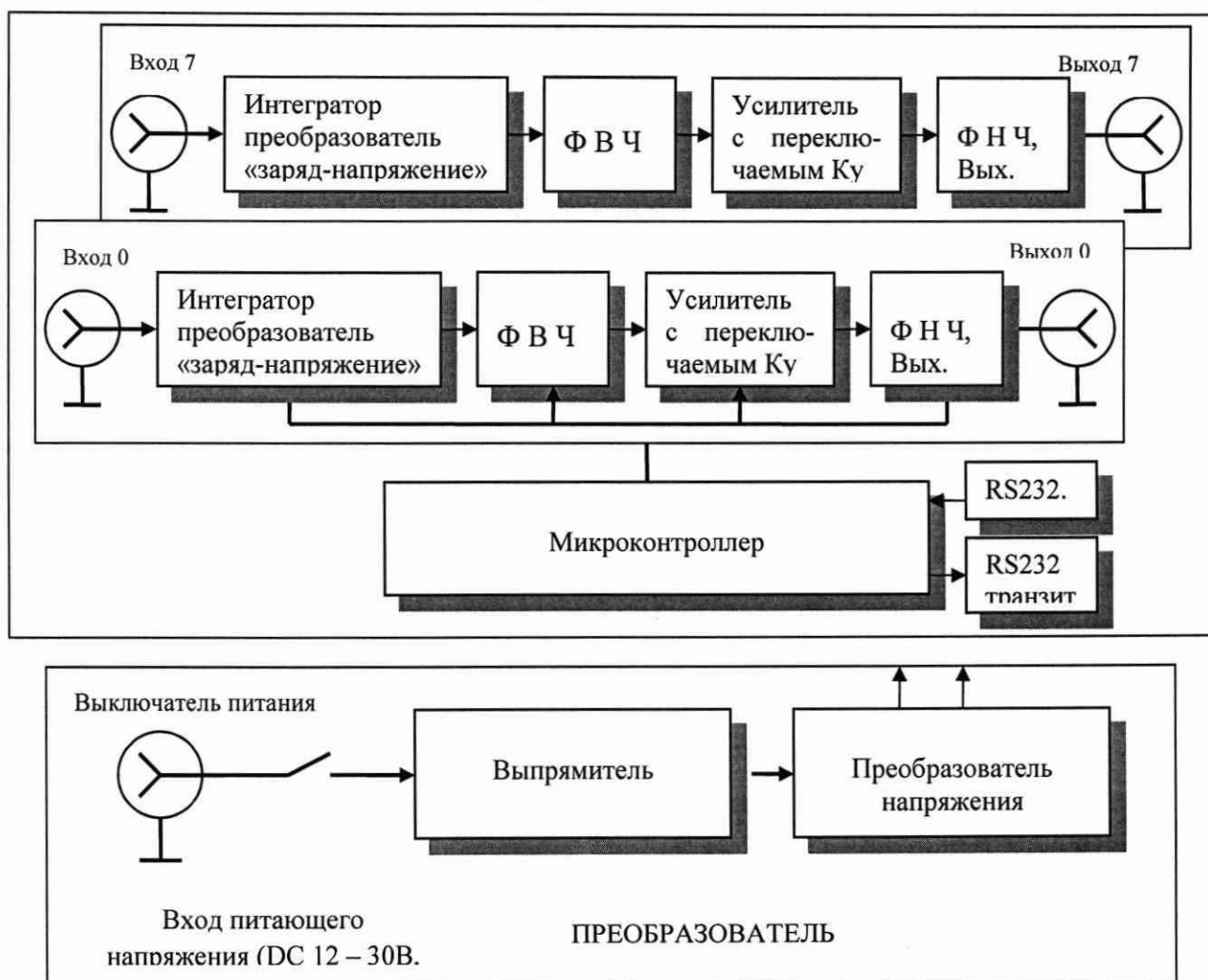
Рисунок 4.3. Структурная схема взаимодействия составных частей РШ2738Э
