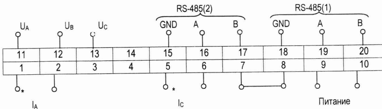
Рисунок А.2 – Двухэлементная трехпроводная схема подключения ЦП 9010
