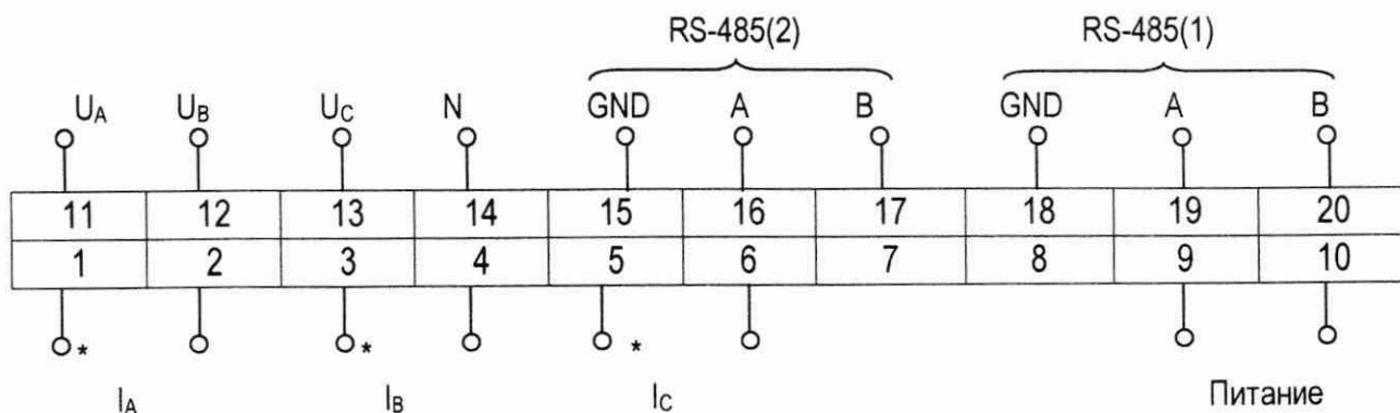
Рисунок А.1 – Трехэлементная четырехпроводная схема подключения ЦП 9010
