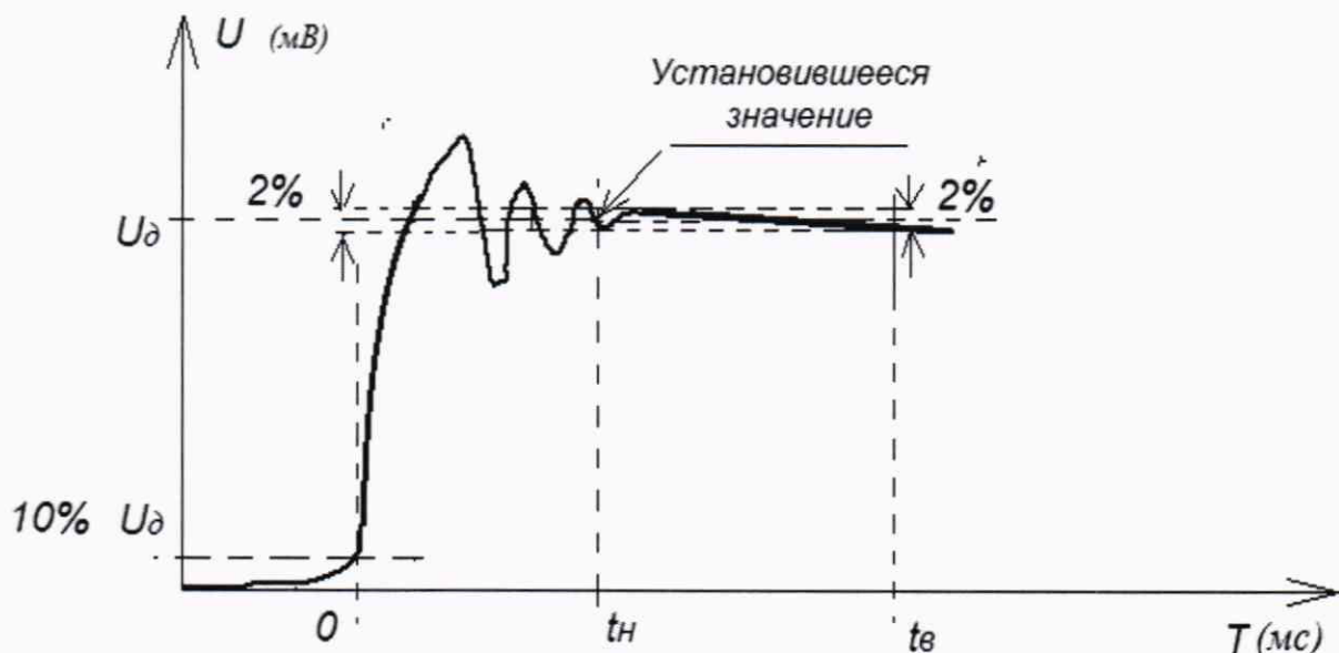
Рисунок 1 - графическое изображение ступени давления
