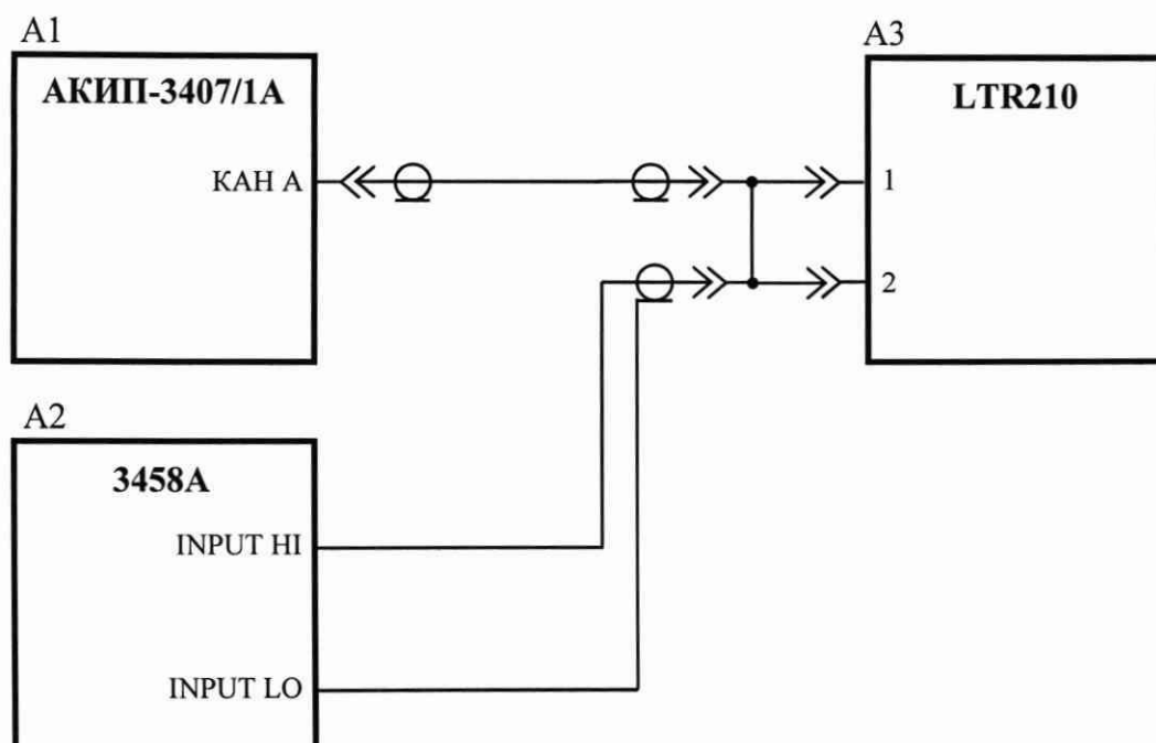
A1 – генератор АКИП-3407/1А; A2 – мультиметр 3458А; A3 – модуль измерительный LTR210.
