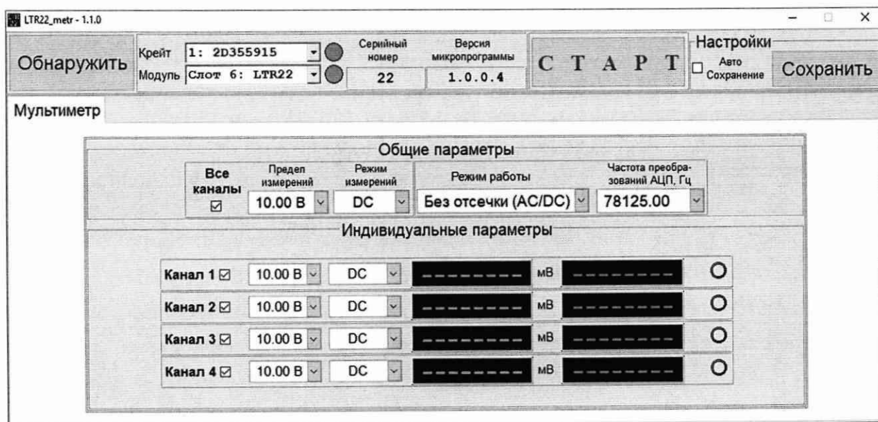
Рисунок 15 – Вид окна программы «LTR22_metr»
