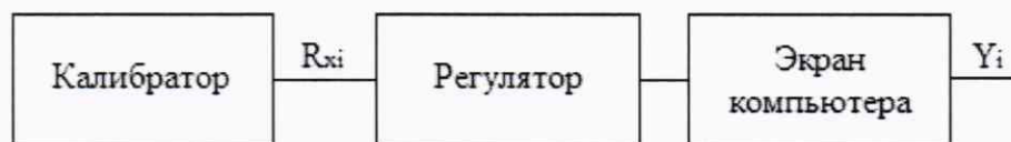
Рисунок 3 - Схема подключений при определении погрешностей ИК, реализующих аналого-цифровое преобразование сигналов от термопреобразователей сопротивления
