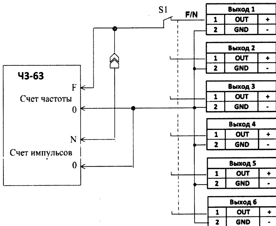
Рисунок А2 – Схема проверки модуля мер частоты (MMC4)
