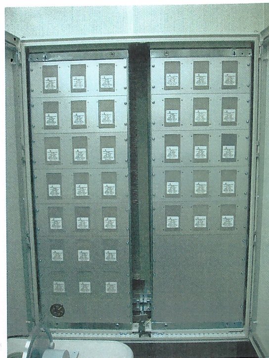
Рисунок 5 - Шкаф кроссовый № 2
