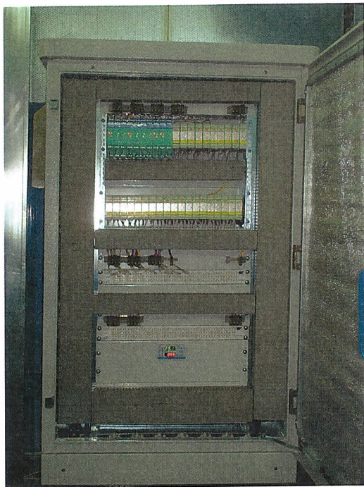
Рисунок 1 - Шкаф термостанционный
