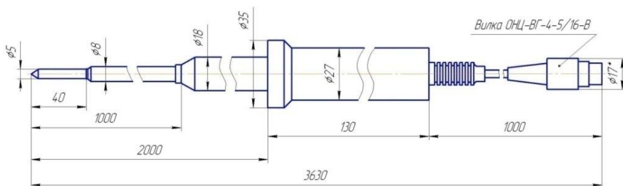
Рисунок 34 – Чертеж общего вида ТСП 9716
