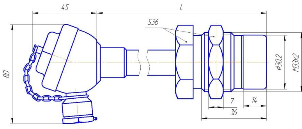
Рисунок 24 – Чертеж общего вида ТСП 9508
