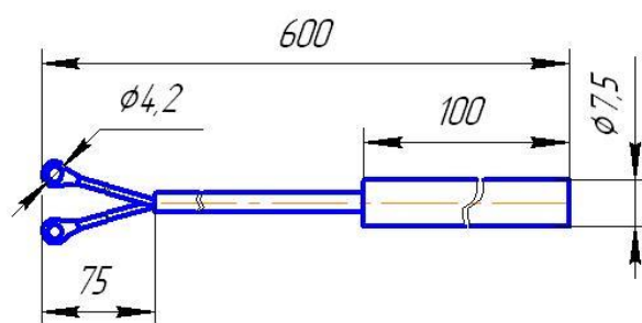
Рисунок 25 – Чертеж общего вида ТСМ 9509
