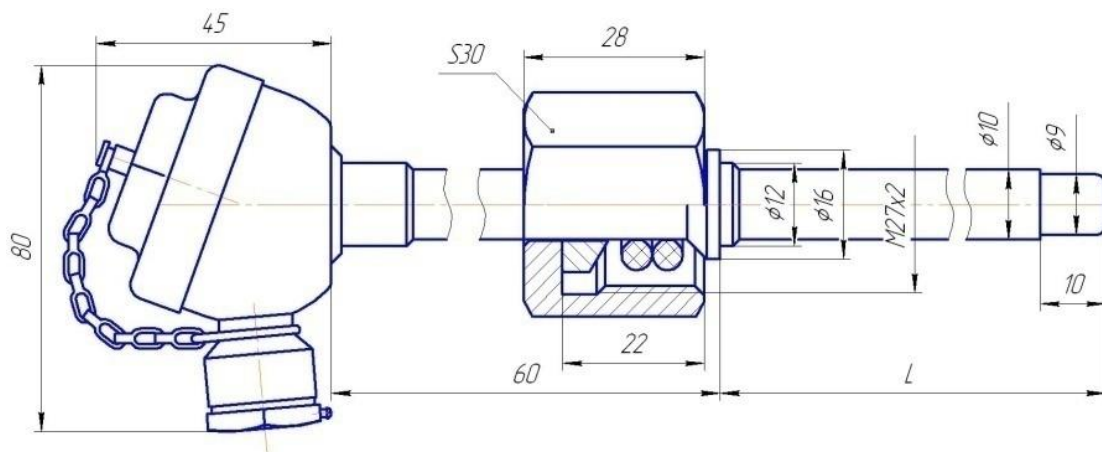
Рисунок 22 – Чертеж общего вида ТСП 9507, ТСМ 9507
