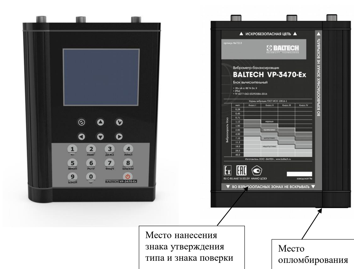
Рисунок 2 - Внешний вид вычислительного блока виброметра BALTECH VP-3470-Ex
