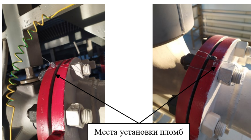
Рисунок 2 – Схема пломбировки от несанкционированного доступа
