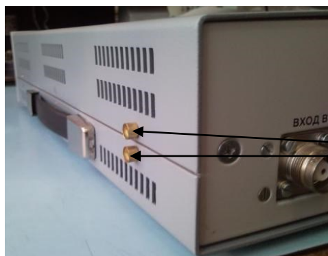
Рисунок 4 – Схема пломбировки приемников от несанкционированного доступа
