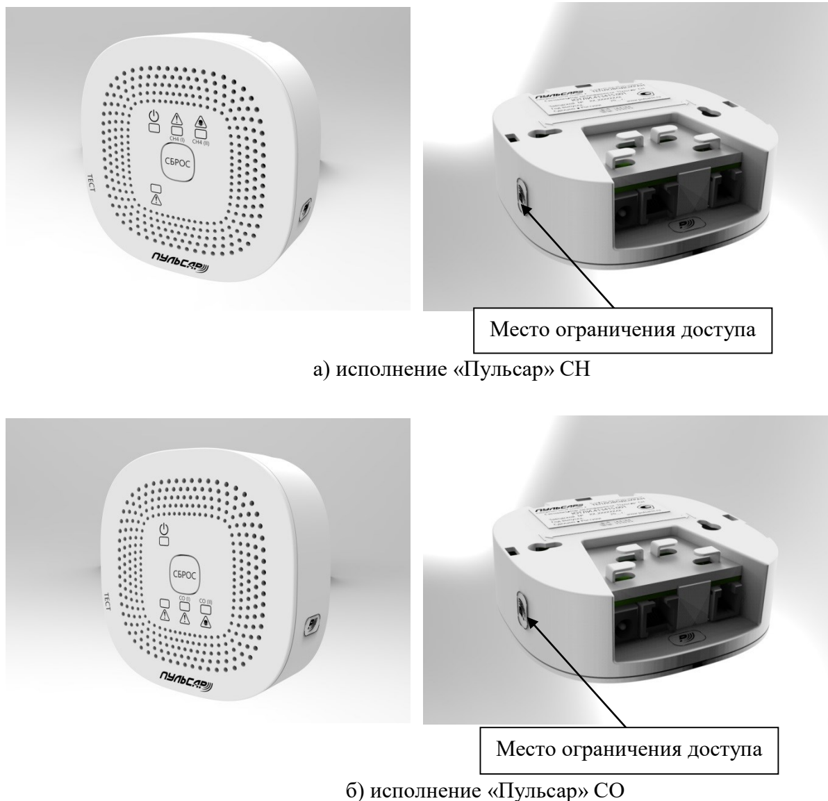
Рисунок 1 - Общий вид сигнализаторов с указанием места ограничения доступа к местам настройки (регулировки)
