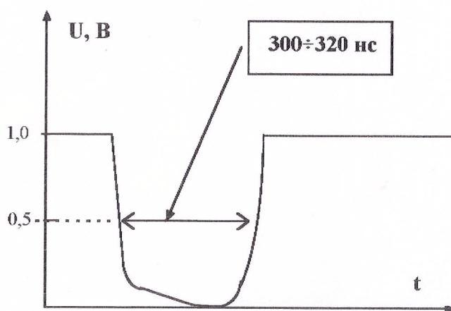
Рис.5. Форма и параметры сигнала 1 Гц на выходе НАП "Грот".
