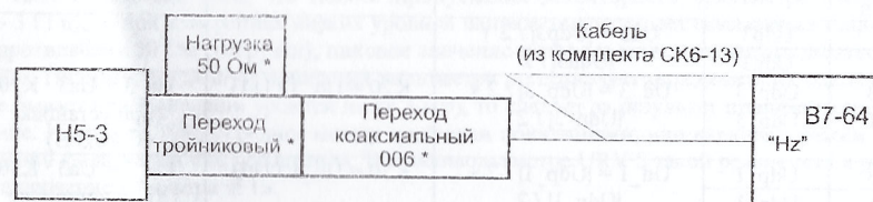
Рисунок 12.3 - Схема для определения погрешности воспроизведения частоты
