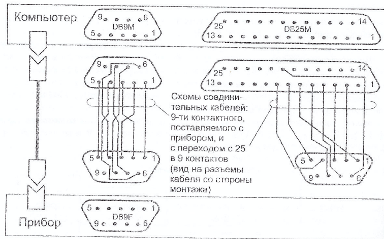
Рисунок 12.5 - Соединение линий интерфейса СТЫК С2 компьютера и прибора
