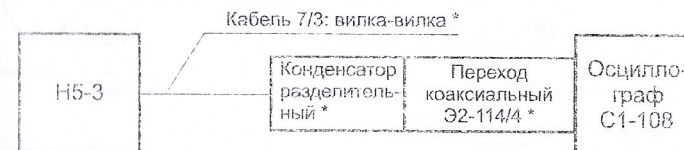
Рисунок 12.4 - Схема для проверки пульсаций в широкой полосе частот
