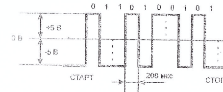
Рисунок 12.6 - Временная диаграмма сигнала на линии
