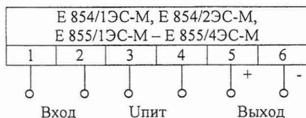
Рисунок Б.1 - Схемы электрические подключений одноканальных ИП
