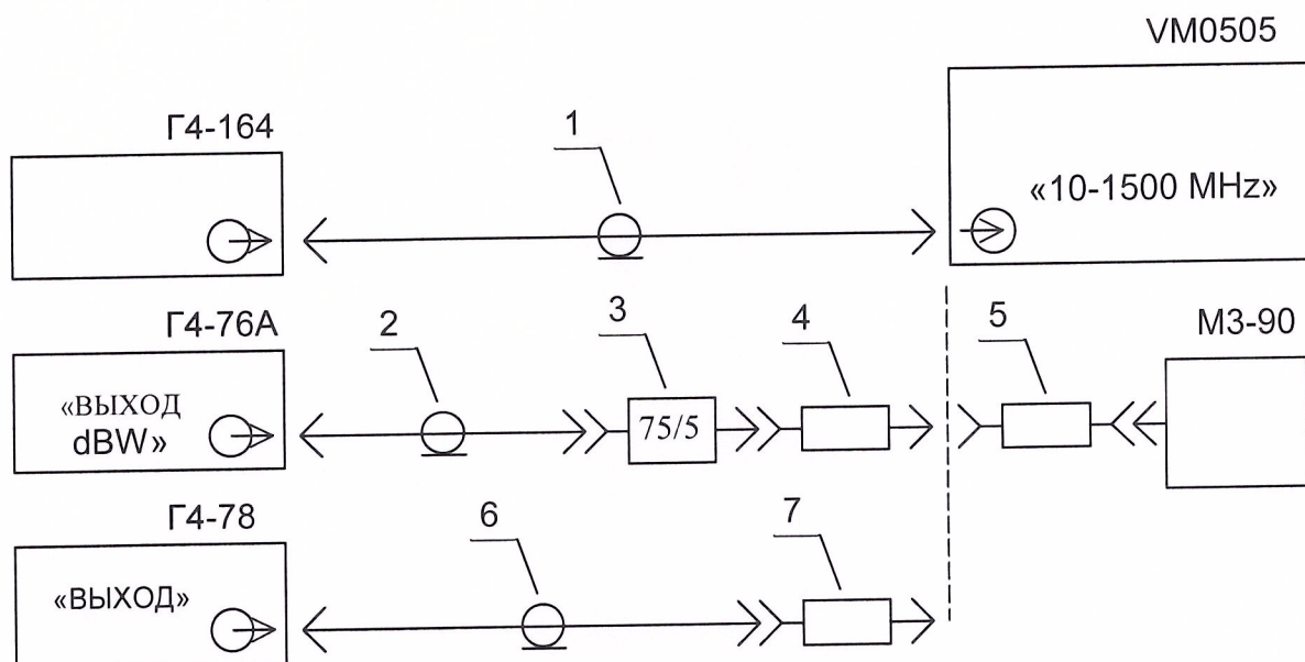
Рисунок 13.3. Схема подключения приборов для проверки неравномерности АЧХ.
