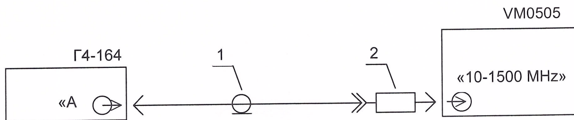
Рисунок 13.5. Схема подключения приборов для проверки гармонических искажений.
