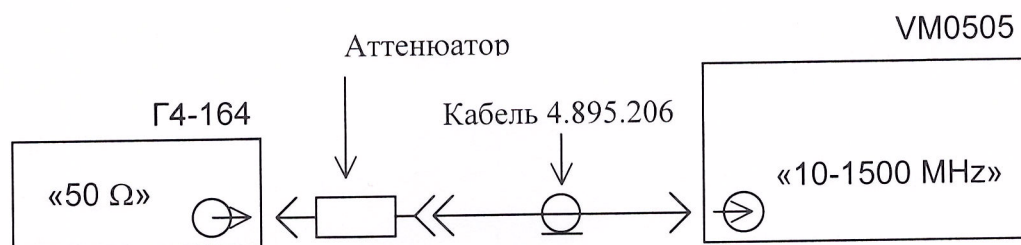
Рисунок 13.2 Схема подключения приборов для проверки погрешности амплитудных шкал.
