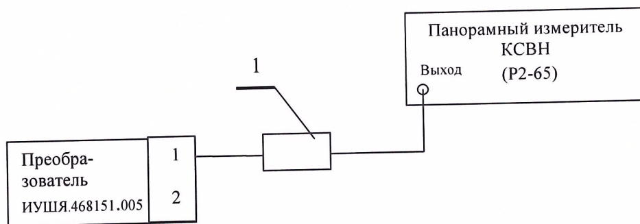
Рисунок 8.5 - Схема подключения приборов при измерении КСВН в диапазоне частот от 18 до 37,5 ГГц
