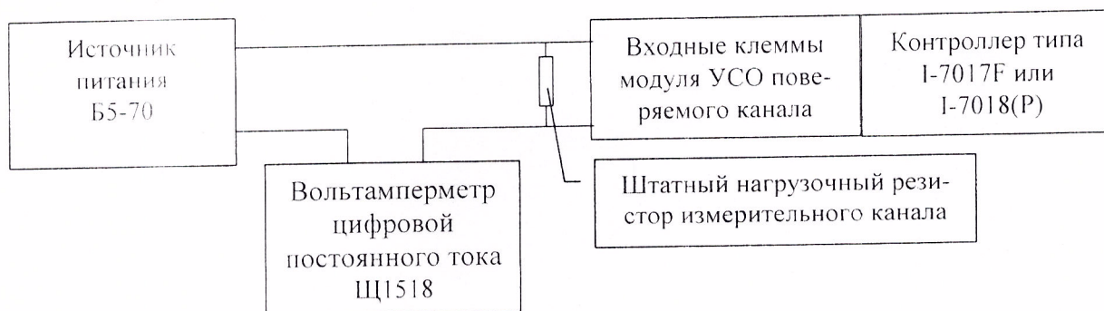
Рис.5. Схема подключения средств испытаний к ИК
