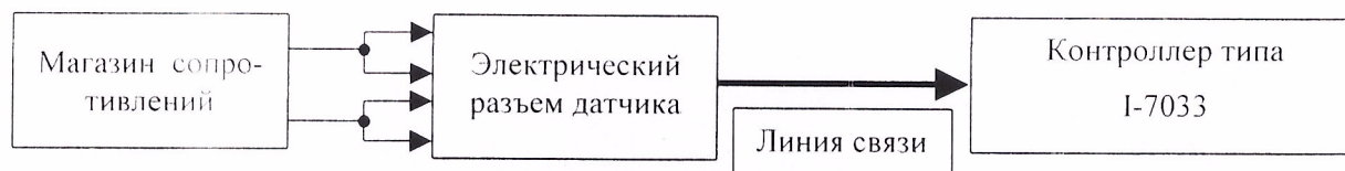
Рис.1. Схема подключения магазина сопротивлений к ИК
