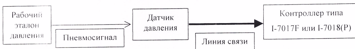
Рис.4. Схема подключения средств испытаний к ИК
